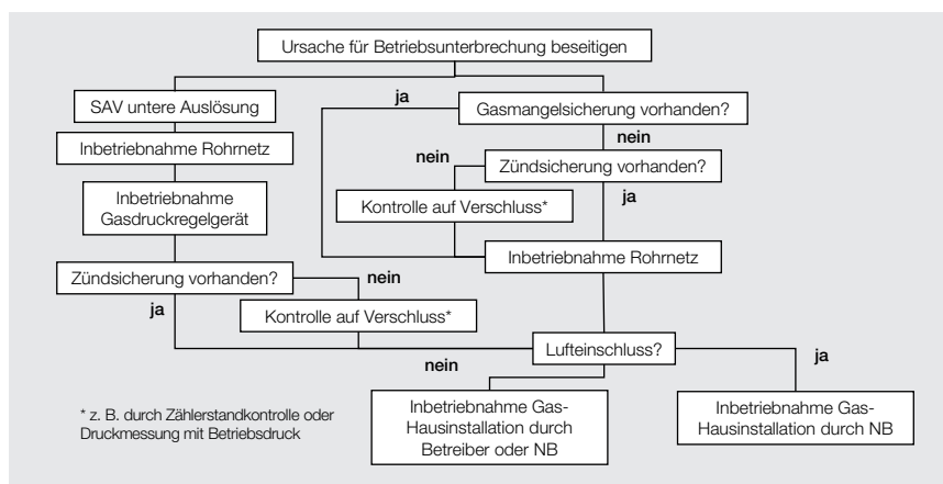
Abb. 2: Ablaufschema zum Vorgang „Einlassen von Gas“
