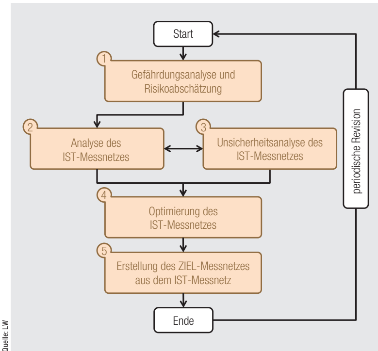
Abb. 3: Schritte zur Optimierung eines Messnetzes
