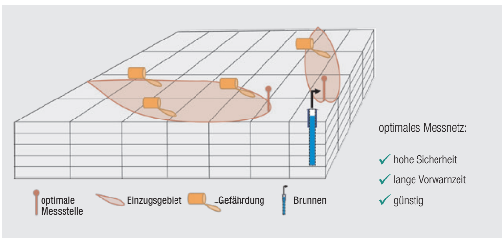
Abb. 2: Beispiel eines optimierten Messnetzes
