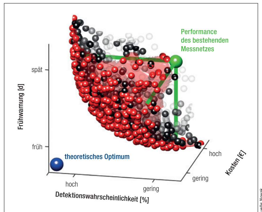
Abb. 5: Pareto-Front (rot) eines multikriteriellen Optimierungsproblems in 3D
