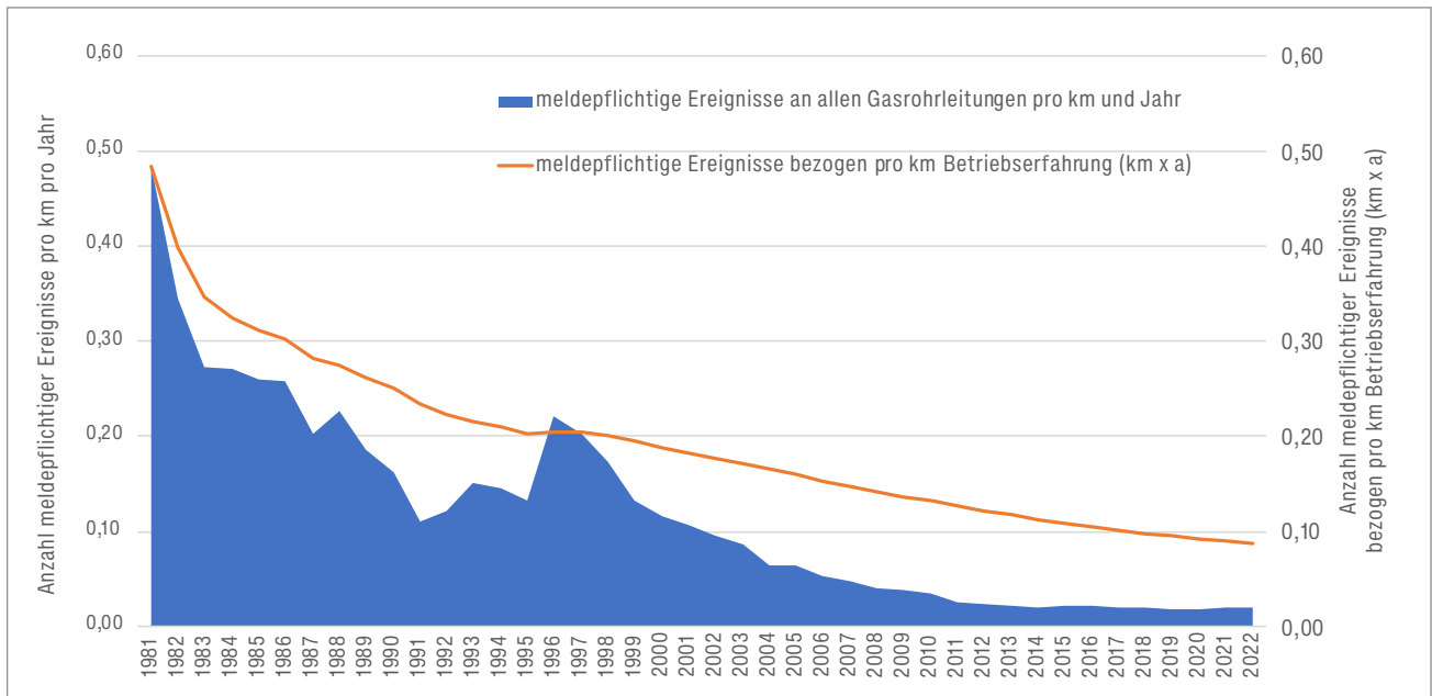
Abb. 11: Entwicklung meldepflichtiger Ereignisse zwischen 1981 und 2022 an allen Gasleitungen
