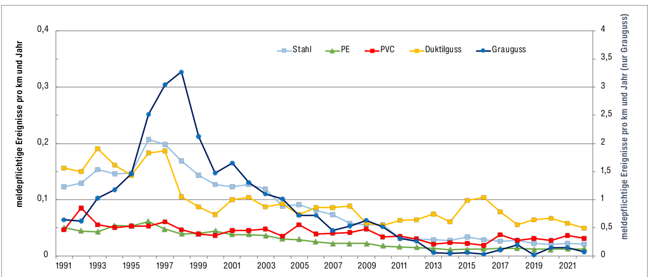
Abb. 12: Entwicklung meldepflichtiger Ereignisse zwischen 1991 und 2022 an allen Gasleitungen nach Werkstoffgruppen
