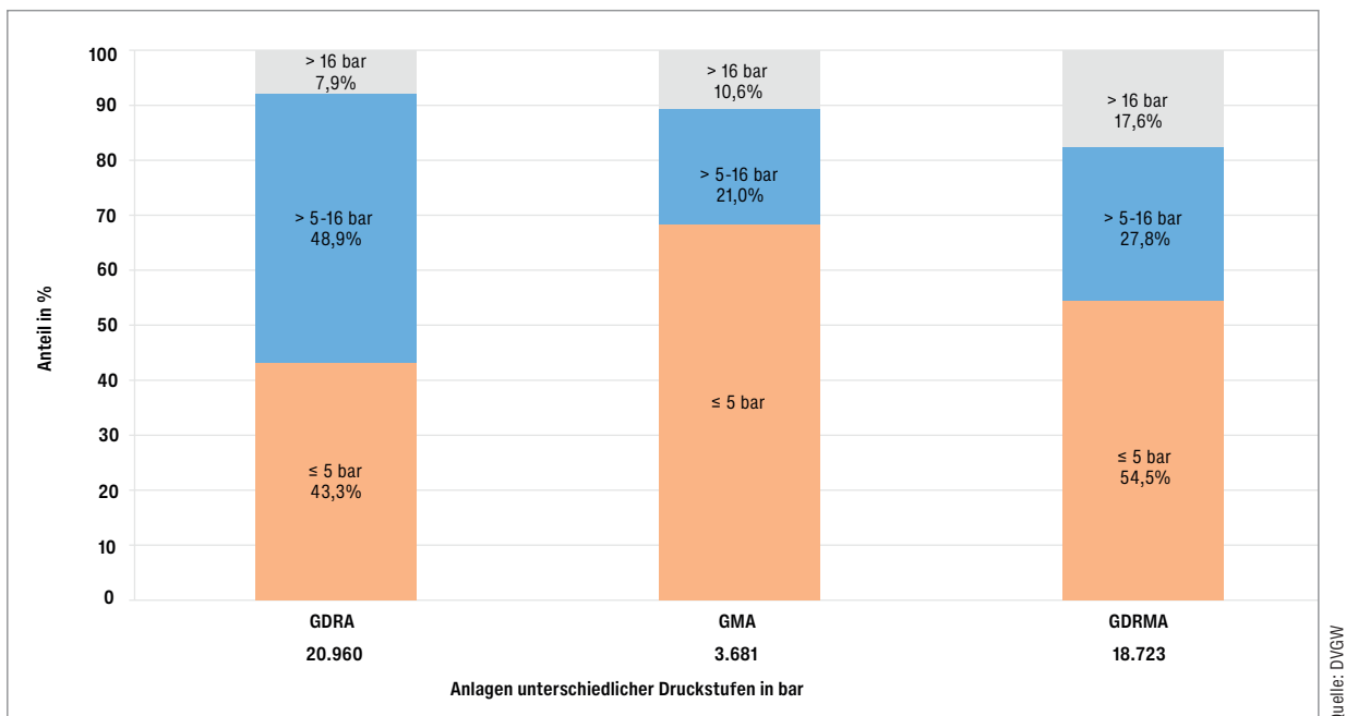
Abb. 10: Anteil von Regel- und/oder Messanlagen unterschiedlicher Druckstufen in Prozent
